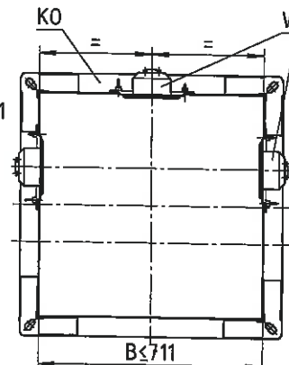
Schnitt A-A Breite B ≤ 711
