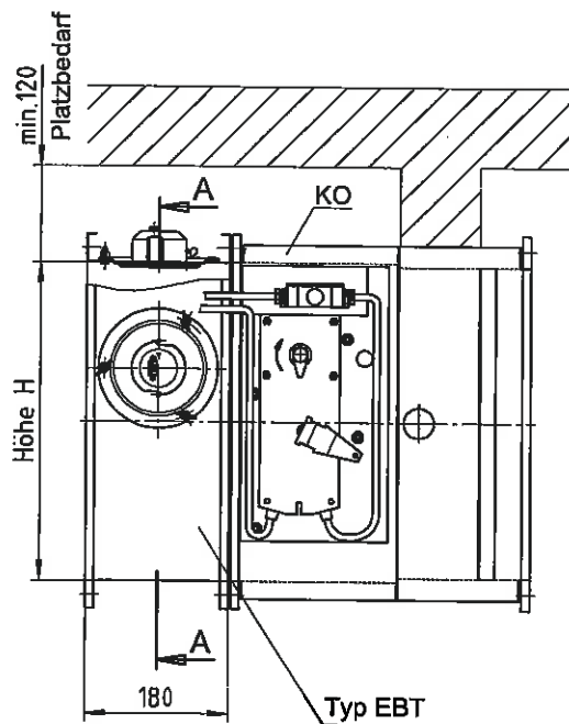
Schnitt A-A Breite B > 711
