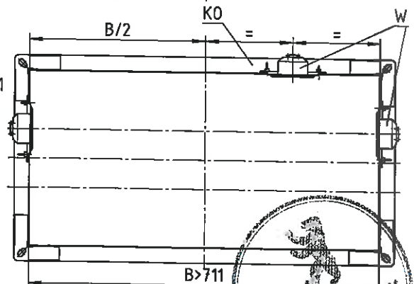
Schnitt A-A Breite B > 711
