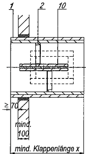
Darstellung ohne Anschlußprofil für Entrauchungsleitung 600° (Stahlblech)
